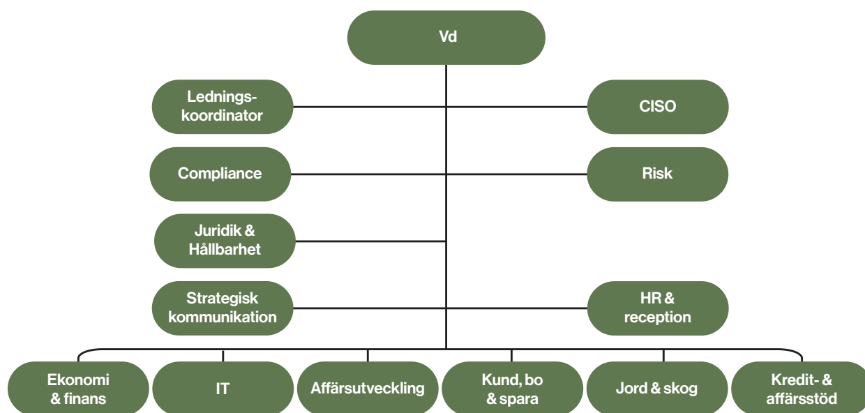
Figur2 Översiktlig organisationsstruktur
