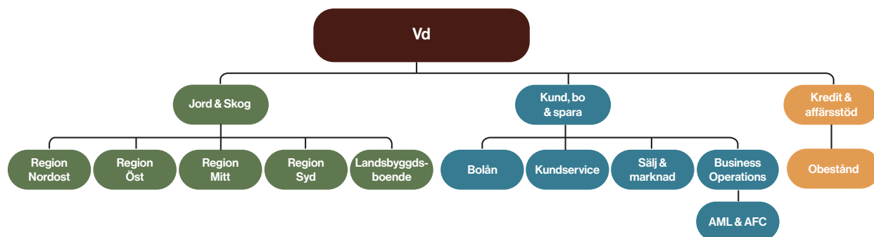
Figur 1 Bankens affärsverksamhet
